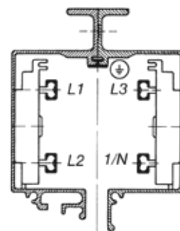
● LSV 5-контактные, 60-300 А
