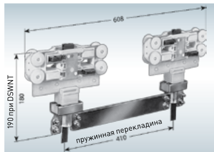
● DSWN 5-контактн., исполнение F
