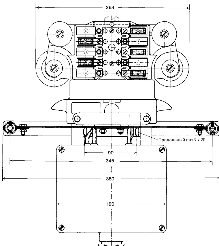
Токоъемник SWNG 11/40 FM с пружинным захватом GFM
