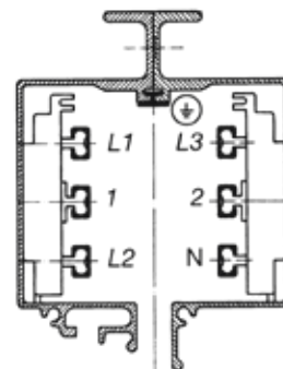
● LSV 6-контактные, 60-200 А
