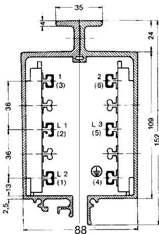
● LSVG 6-контактные, 60-300 А
