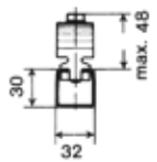
Позиция прихвата для D = 15-25 мм
