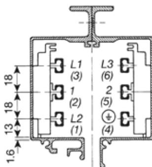
● LSV 5-контактные, 60-200 А
